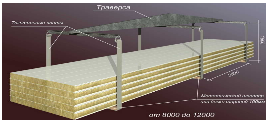
Рисунок 10 – Схема строповки пакетов панелей длиной более 8000 мм
