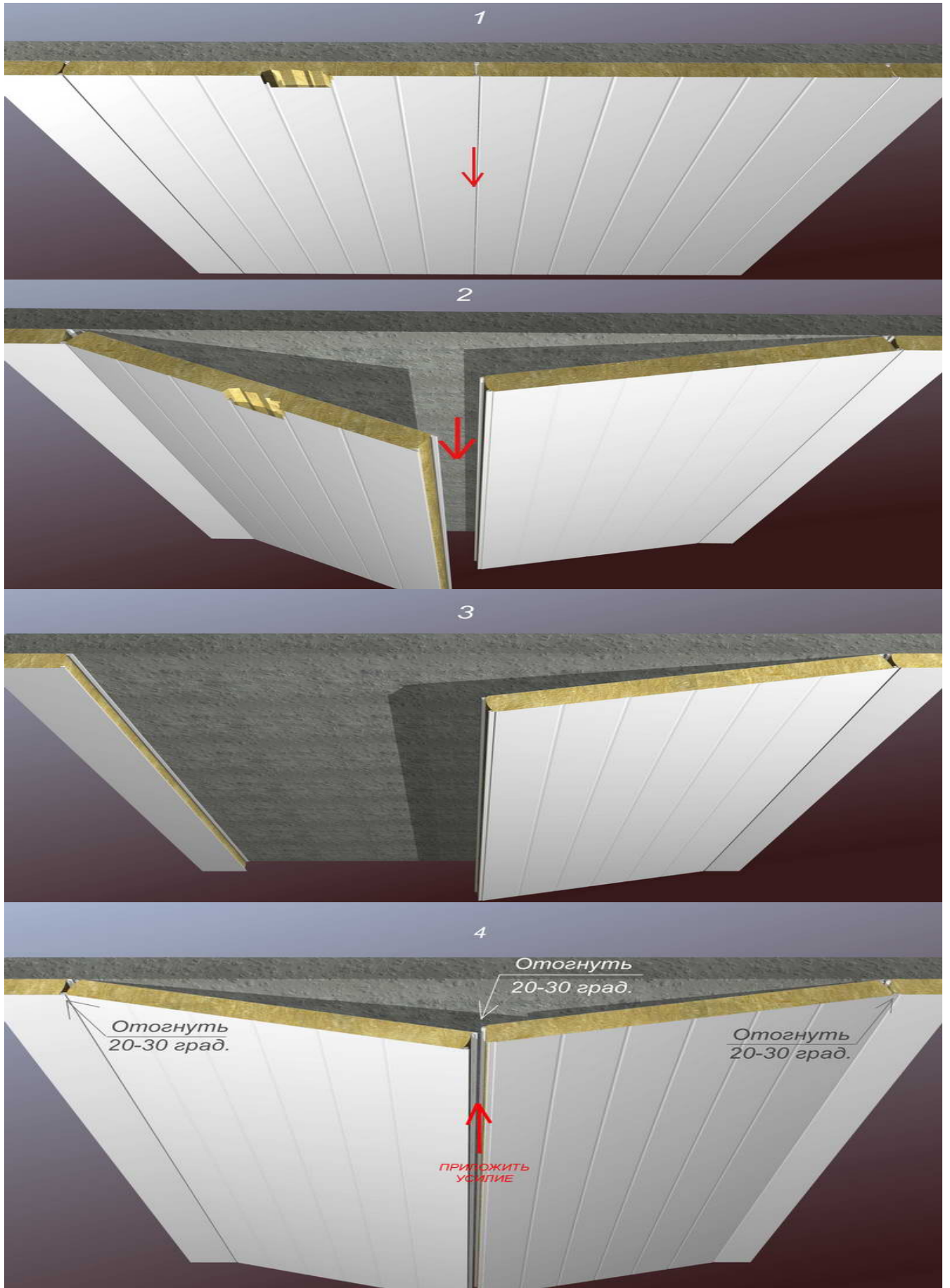
Рисунок 14 – Замена поврежденных стеновых панелей
