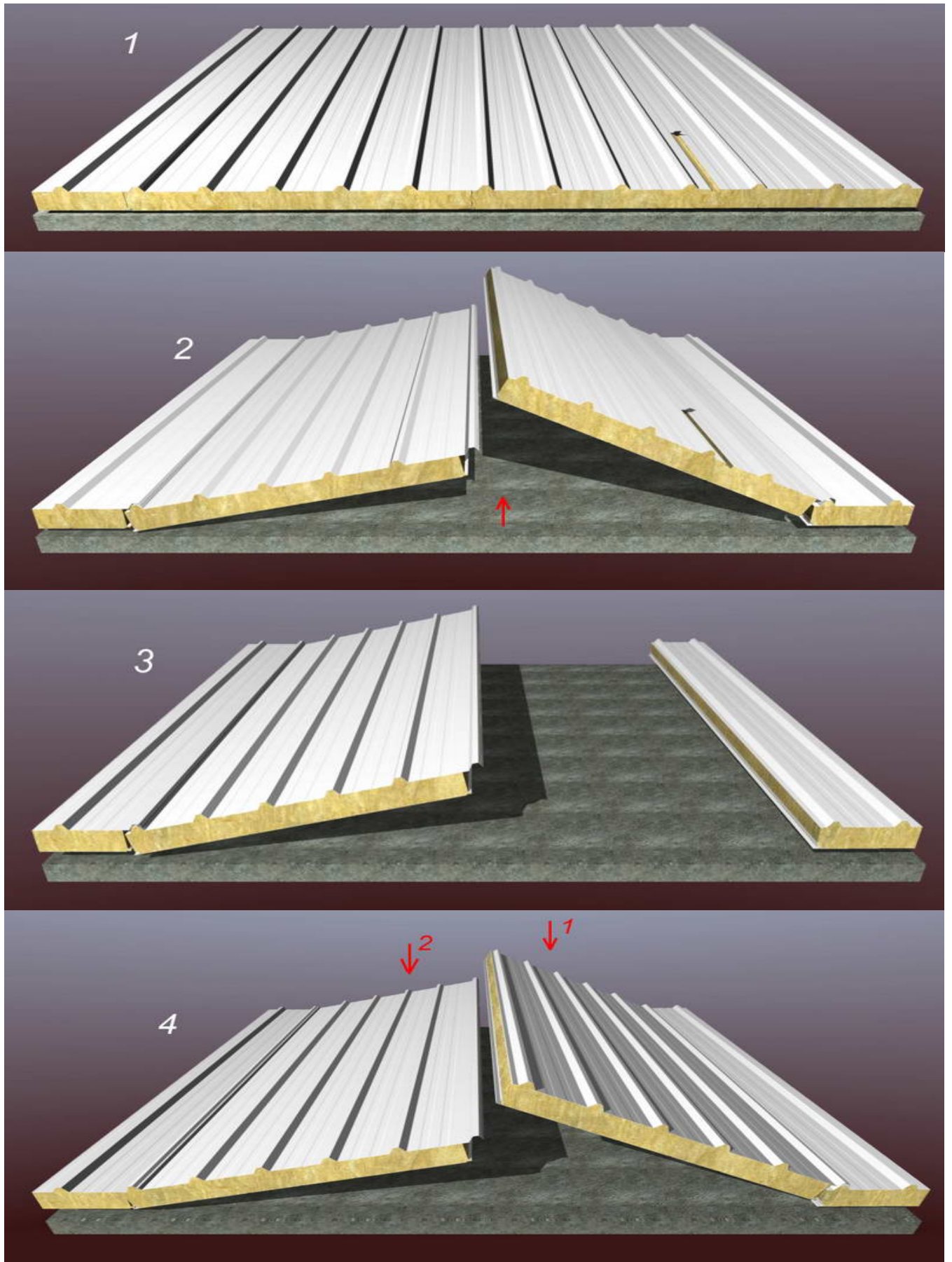
Рисунок 15 – Замена поврежденных кровельных панелей
