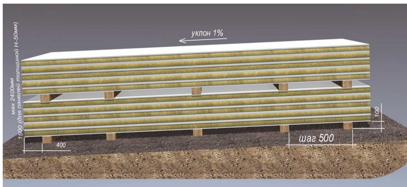
Рисунок 11 – Схема складирования пакетов панелей
