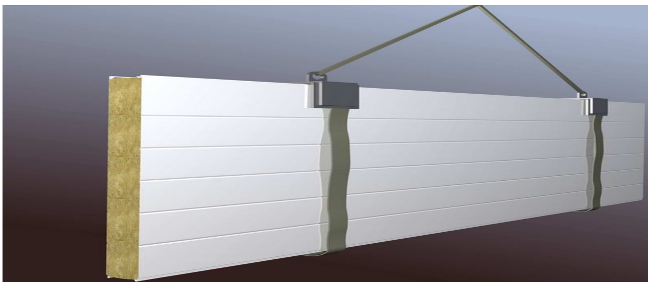
Рисунок 12б – Подвеска стеновых панелей при горизонтальном перемещении с помощью управляющего троса
